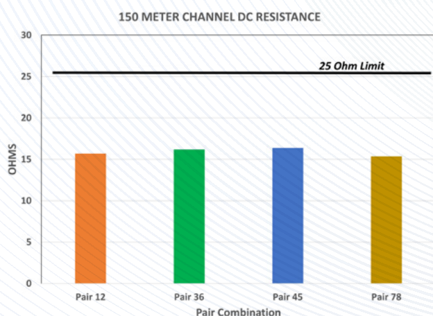
図 14: 150 m チャンネルの DC 抵抗 (140 m の 22 AWG Cat6 ケーブル、および 10 m の 24 AWG Cat6 パッチコード)
