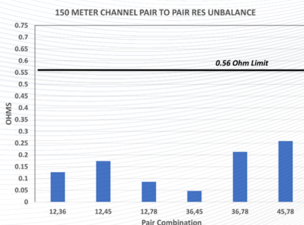
図 16: 150 m チャンネルのペア間の抵抗のアンバランス (140 m の 22 AWG Cat6 ケーブル、および 10 m の 24 AWG Cat6 パッチコード)
