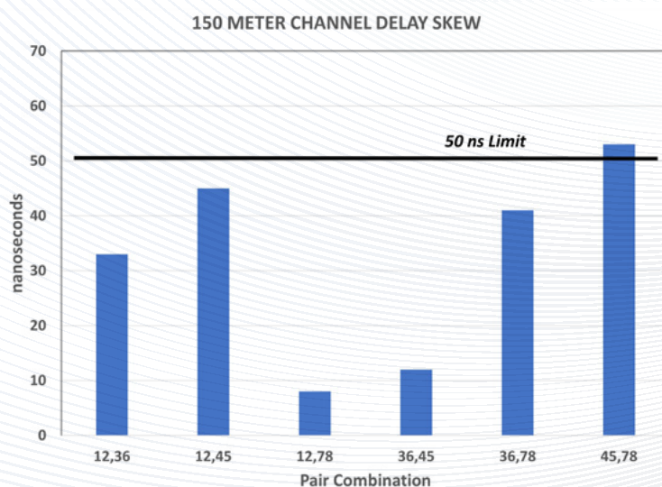
図 13: 150 m チャネルの遅延時間差 (140 m の 22 AWG Cat6 ケーブル、および 10 m の 24 AWG Cat6 パッチコード)
