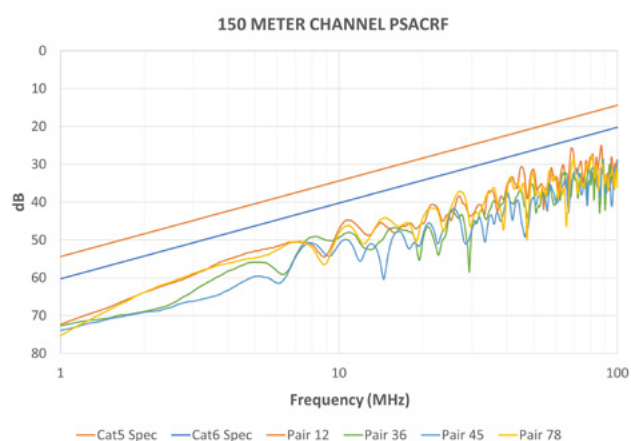
図 11: 150 m チャンネルの PSACRF (140 m の 22 AWG Cat6 ケーブル、および 10 m の 24 AWG Cat6 パッチコード)
