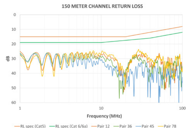
図 12: 150 m チャンネルの反射減衰量 (140 m の 22 AWG Cat6 ケーブル、および 10 m の 24 AWG Cat6 パッチコード)
