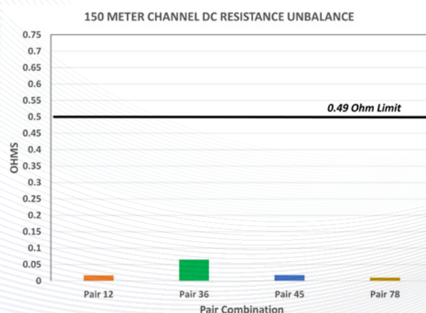
図 15: 150 m チャンネルの抵抗アンバランス (140 m の 22 AWG Cat6 ケーブル、および 10 m の 24 AWG Cat6 パッチコード)
