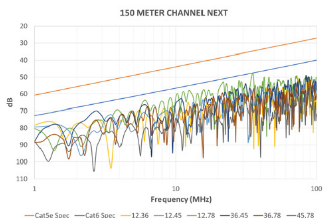
図 10: 150 m チャンネルの NEXT (140 m の 22 AWG Cat6 ケーブル、および 10 m の 24 AWG Cat6 パッチコード)
