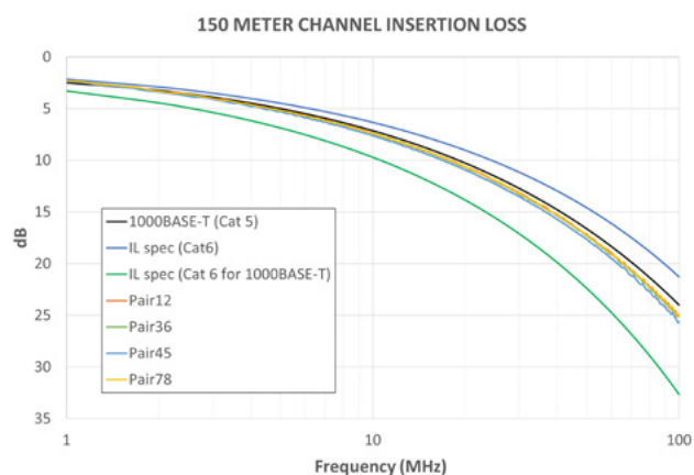
図 9: 150 m チャンネルの挿入損失 (140 m の 22 AWG Cat6 ケーブル、および 10 m の 24 AWG Cat6 パッチコード)
